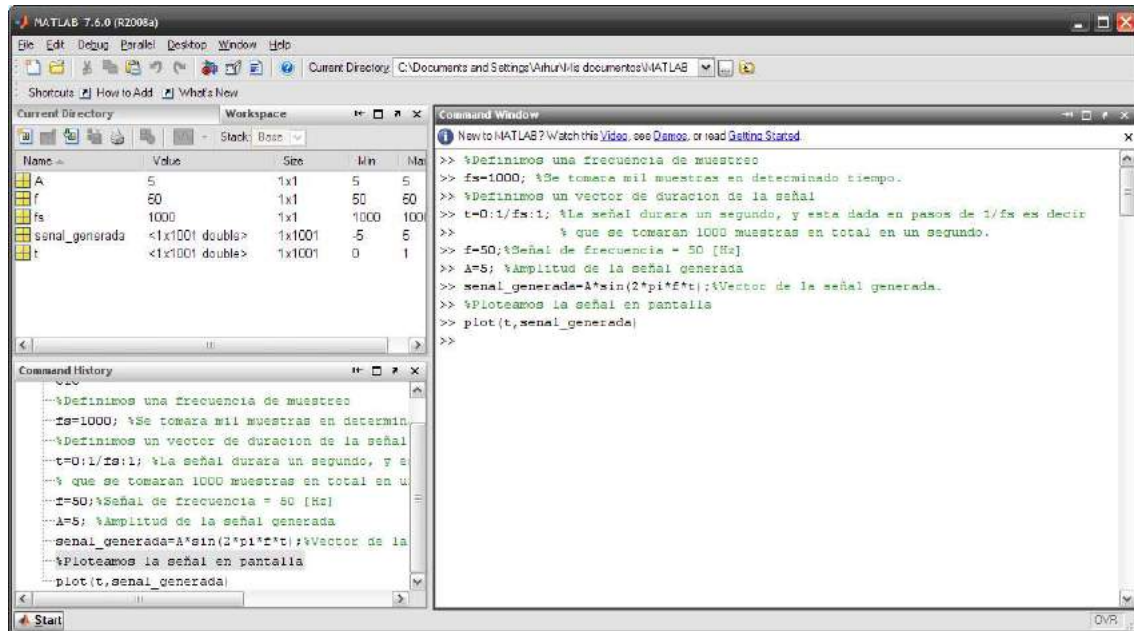
Figura 3: Código de una función sinusoidal
