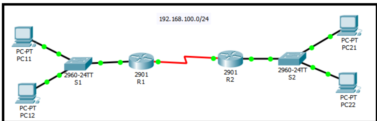
Figura 1. Topología de red, enlace WAN con HDLC
